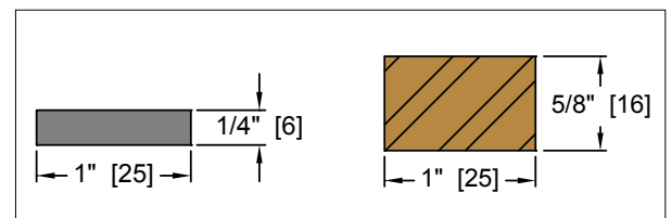
EXTERIOR MUNTIN
