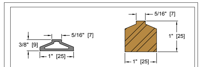
EXTERIOR MUNTIN
