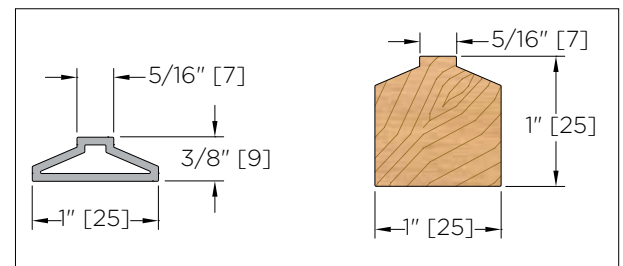
EXTERIOR MUNTIN
